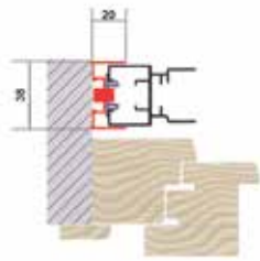
Magnetprofil*
