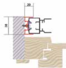
Montageprofil*
